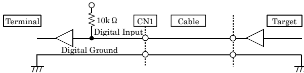
図3.7 デジタル入力の接続
