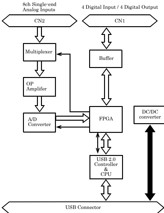
図7.2 回路ブロック図
