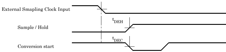
図7.3 外部サンプリングクロックのタイミング
