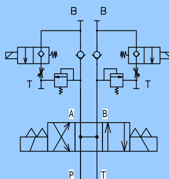
圧力保持回路
